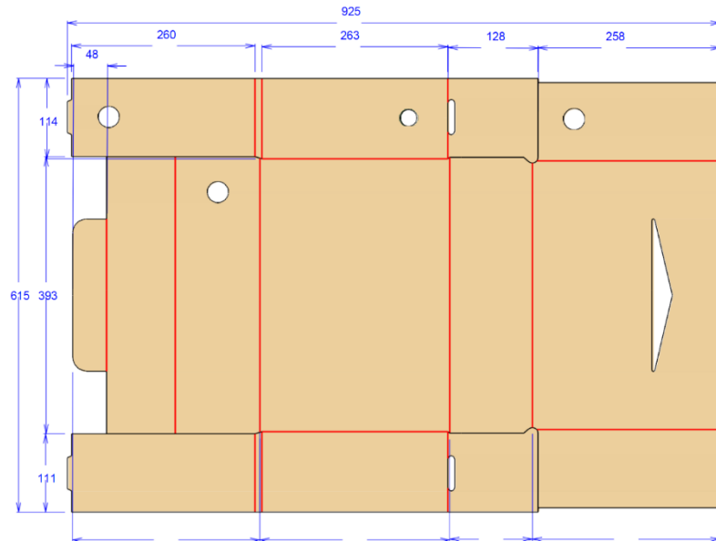
DIMENSIONES CAJA TIPO MALETIN: Las dimensiones están expresadas en milímetros.
