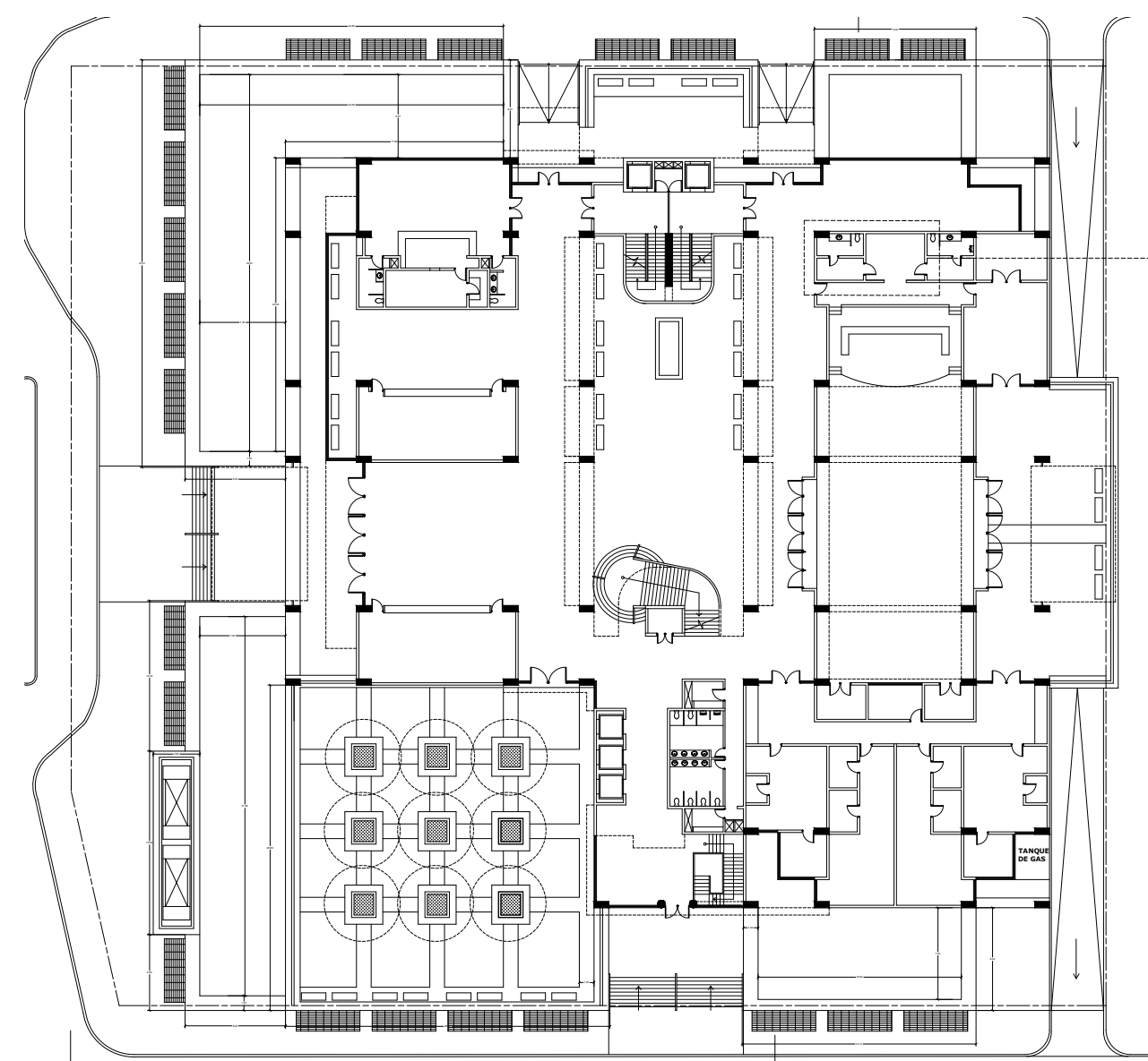
Planta arquitectónica 1er nivel
