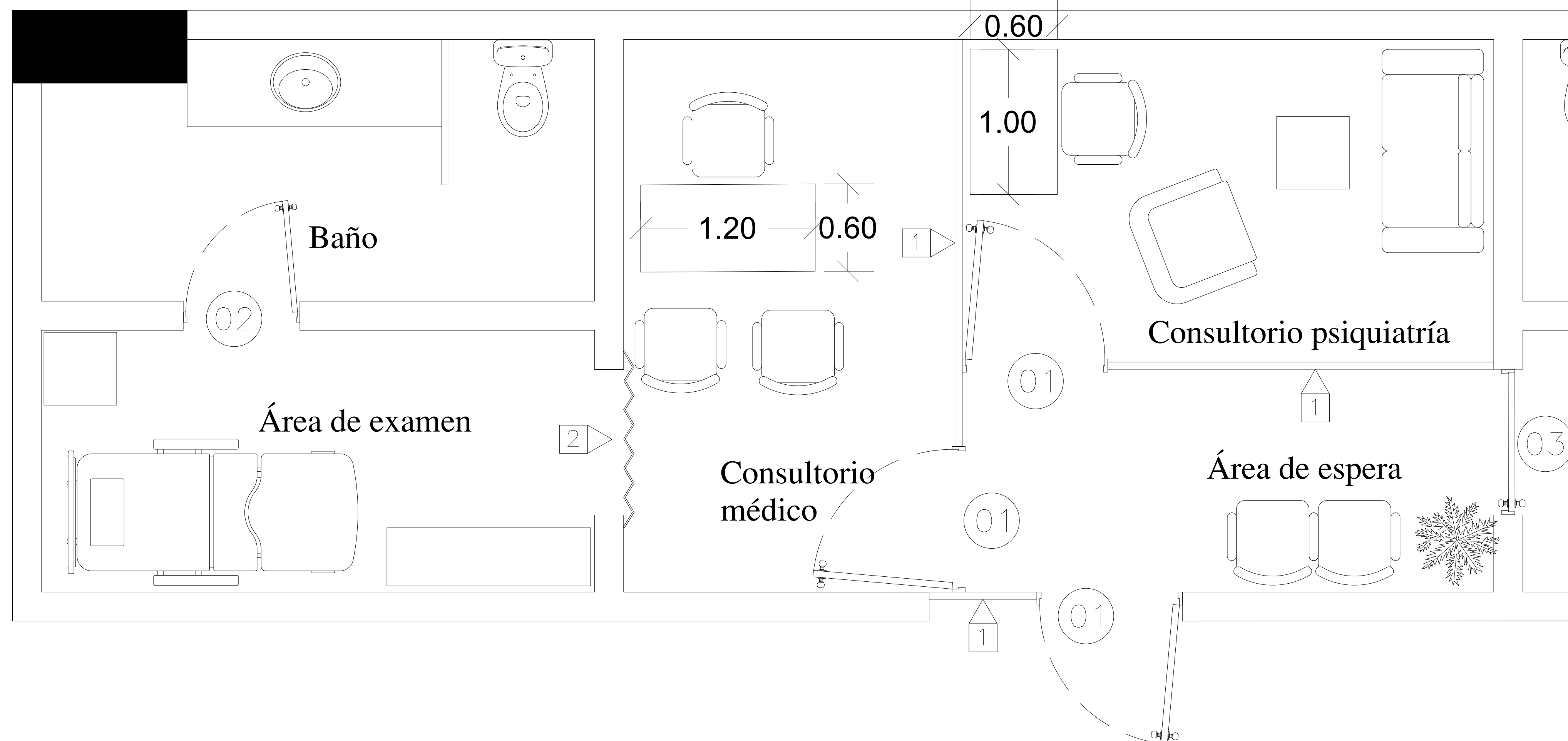
Planta arquitectonica propuesta ESCALA: 1:20
