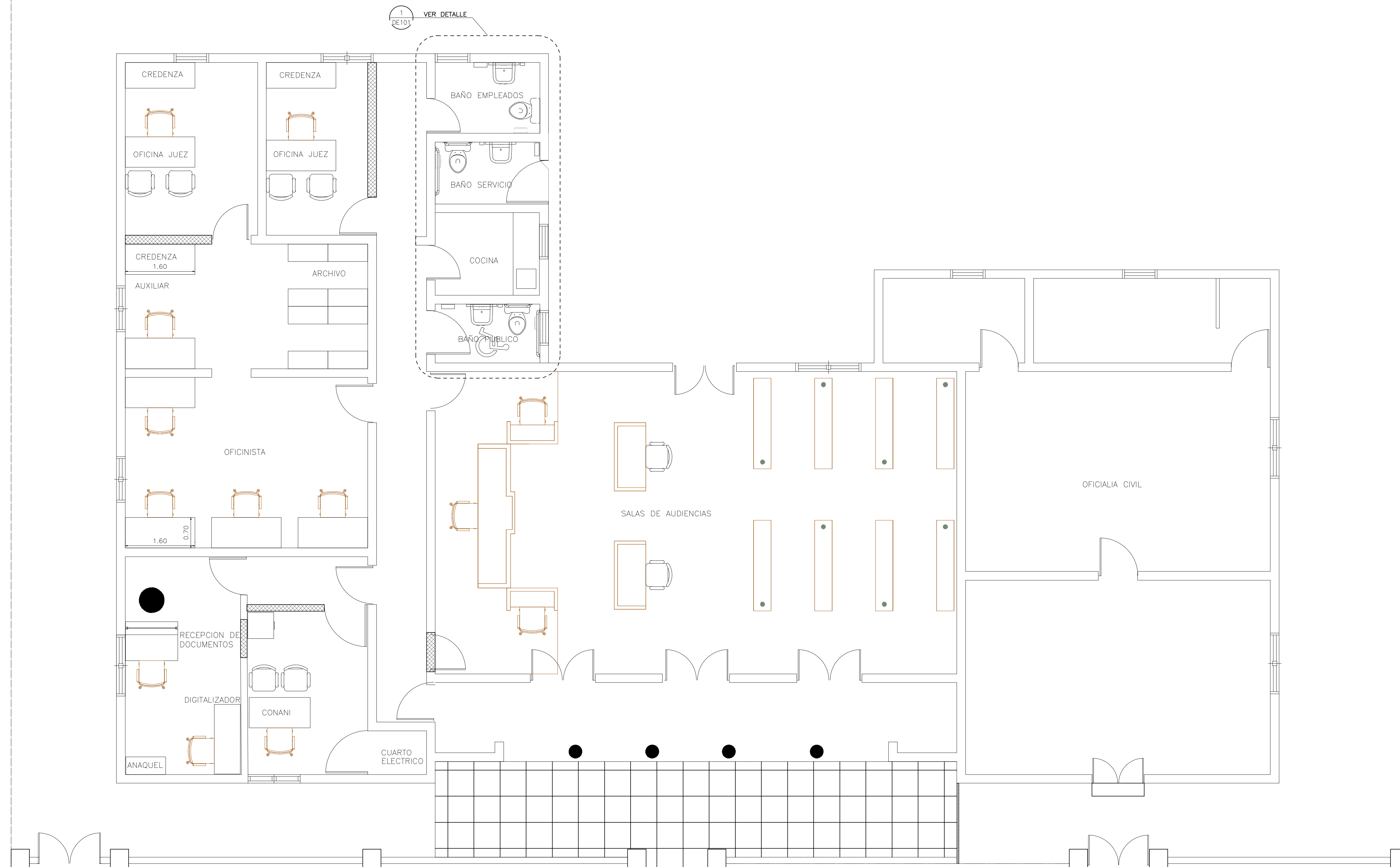
PLANTA ARQUITECTONICA PROPUESTA TRIBUNAL NNA ESCALA: 1:50
