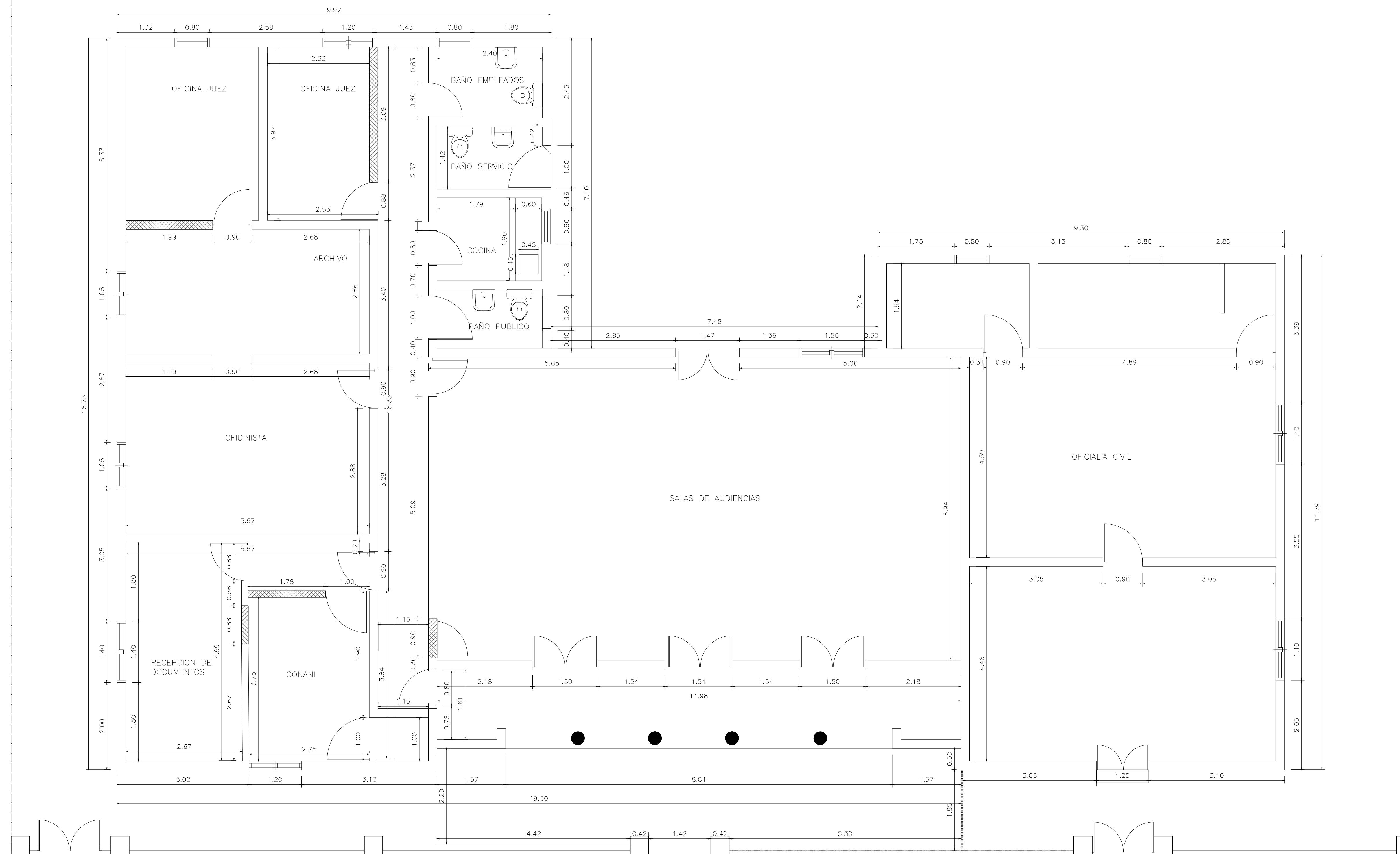
PLANTA DIMENSIONADA PROPUESTA TRIBUNAL NNA ESCALA: 1:50
