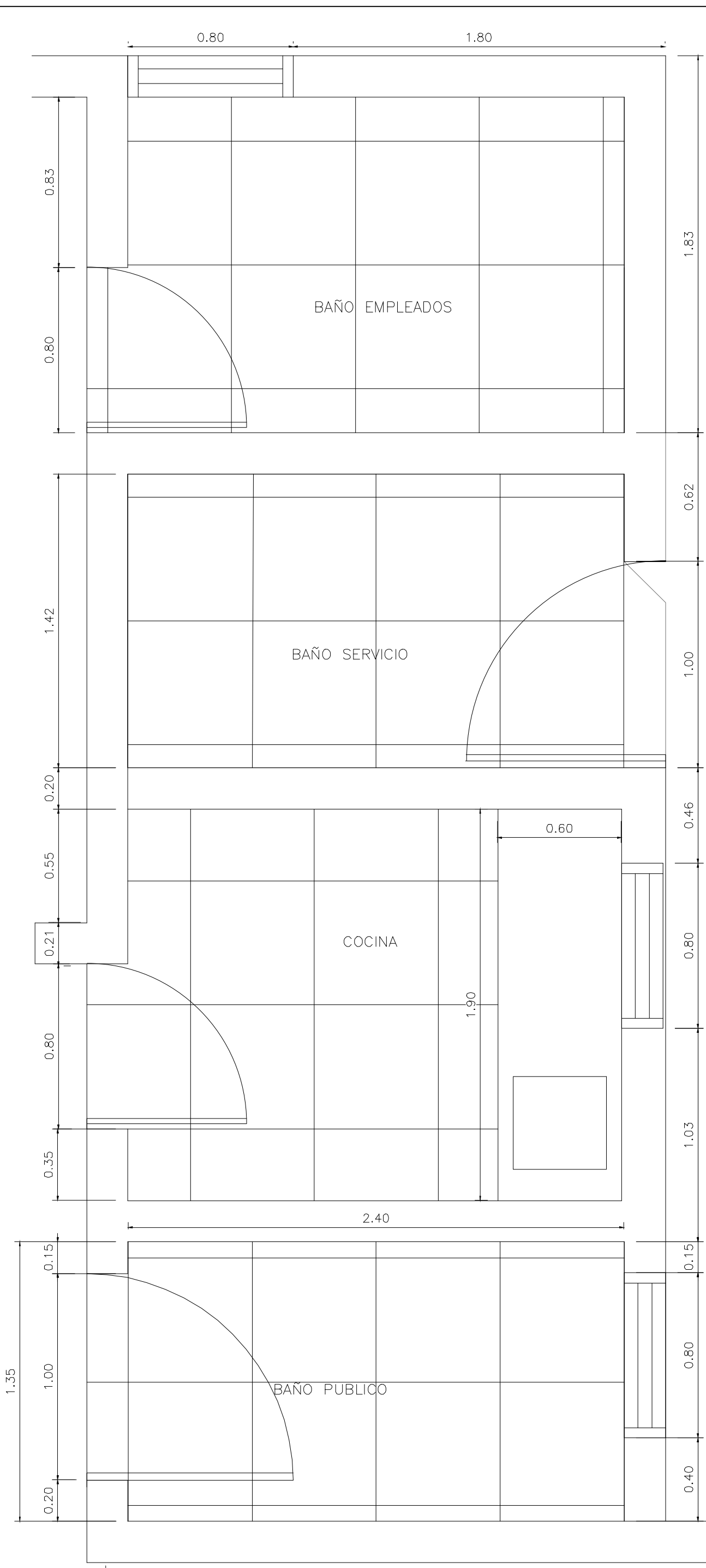
PLANTA PROPUESTA DE PISOS
