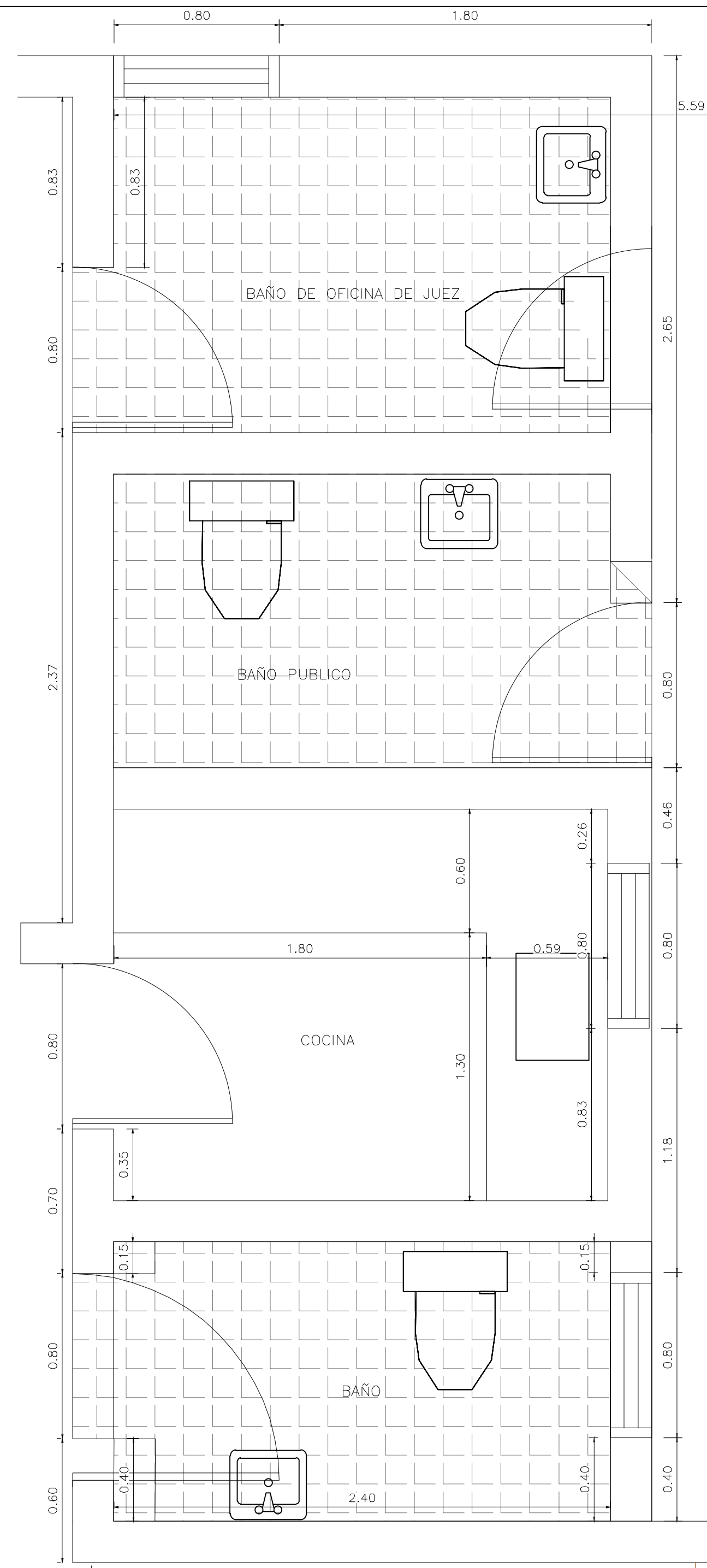
PLANTA EXISTENTE DE BAÑOS Y COCINA
