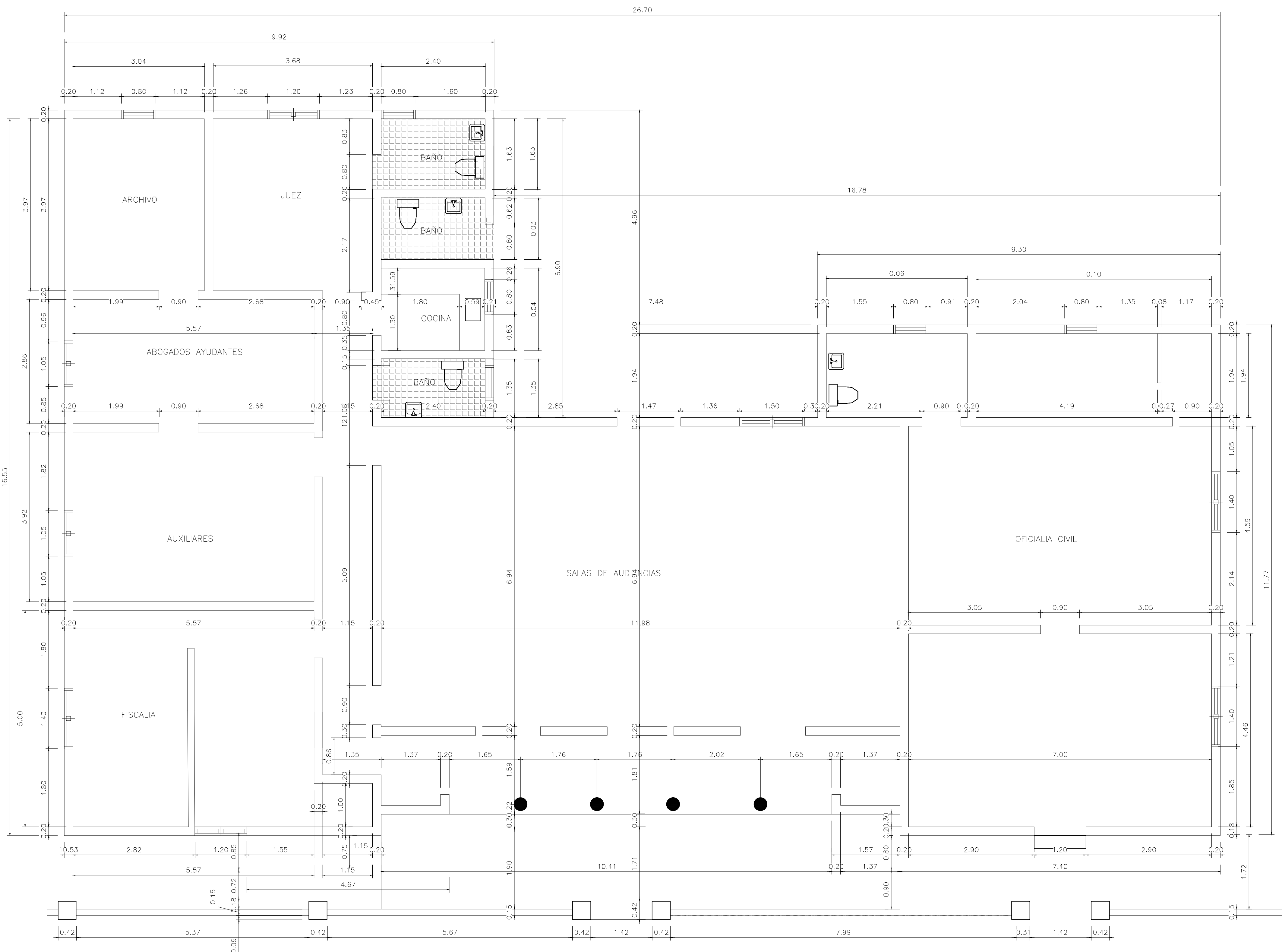
PLANTA DIMENSIONADA 1ER NIVEL ESCALA: 1:75
