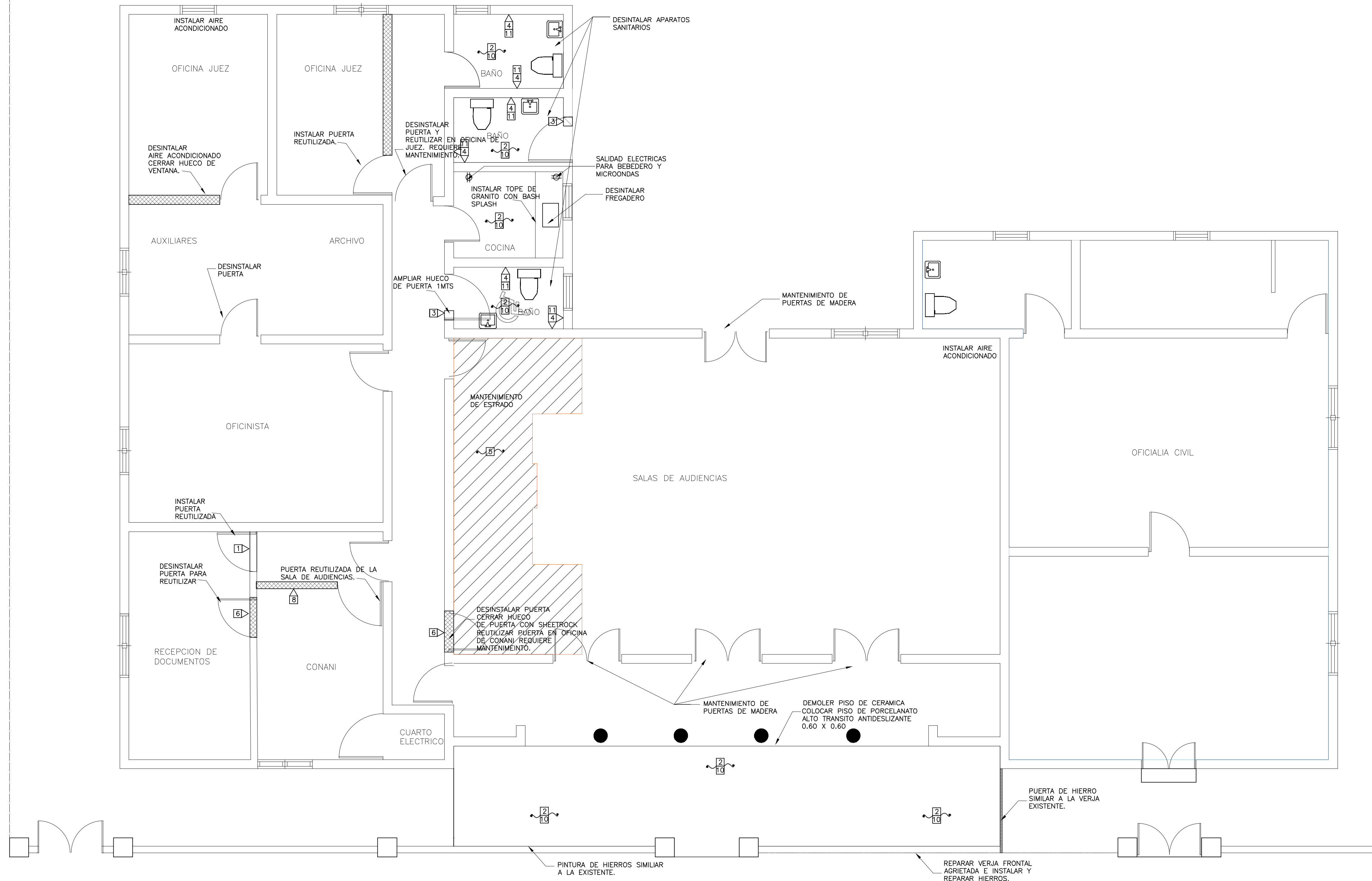
PLANTA ARQUITECTONICA DE INTERVENCIONES CONSTRUCTIVAS ESCALA: 1:50
