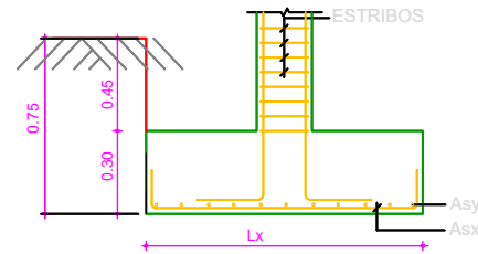
SECCIÓN ZAPATA COLUMNAS
