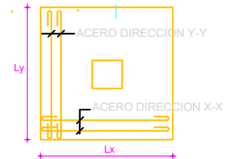
PLANTA DE ZAPATA Z1
