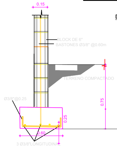
SECCION A-A' ZAPATA DE MUROS DE MAMPOSTERIA
