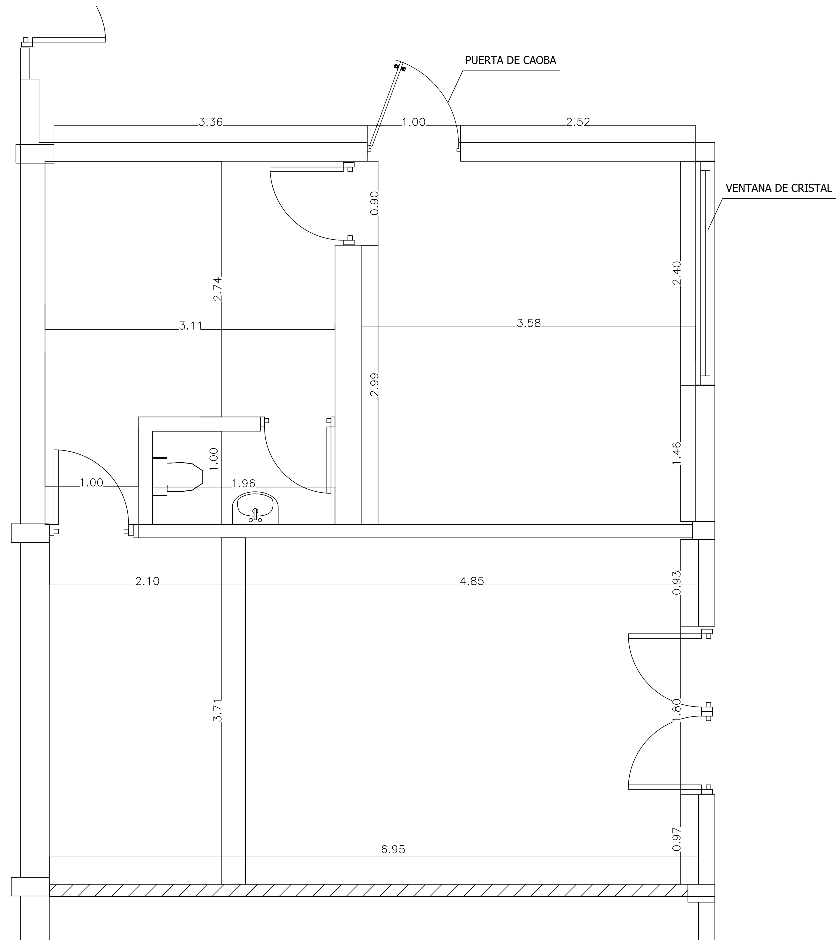
PLANTA ARQUITECTONICA DIMENSIONADA ESCALA: 1:50
