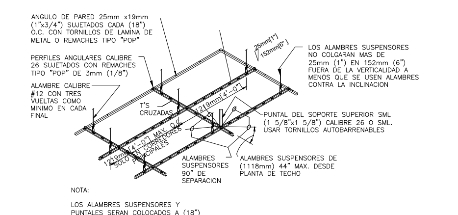
DETALLE TIPICO INSTALACION DE TECHO SUSPENDIDO ESCALA: NO A ESCALA
