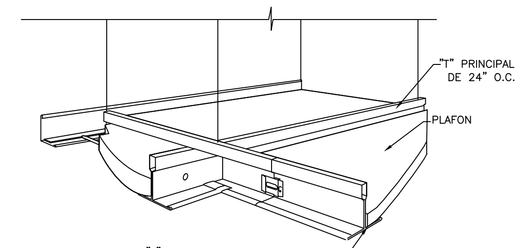
SISTEMA PLAFON SUSPENDIDO ESCALA: NO A ESCALA
