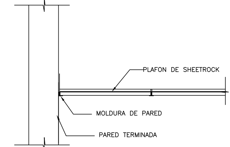
SISTEMA PLAFON SUSPENDIDO ESCALA: NO A ESCALA
