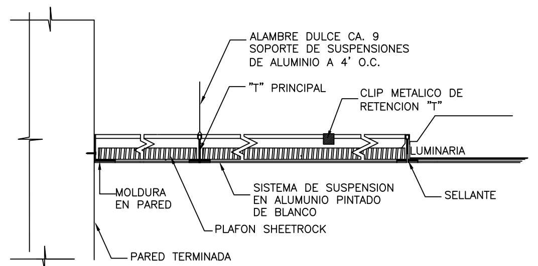
DETALLE INSTALACION PLAFON ESCALA: NO A ESCALA
