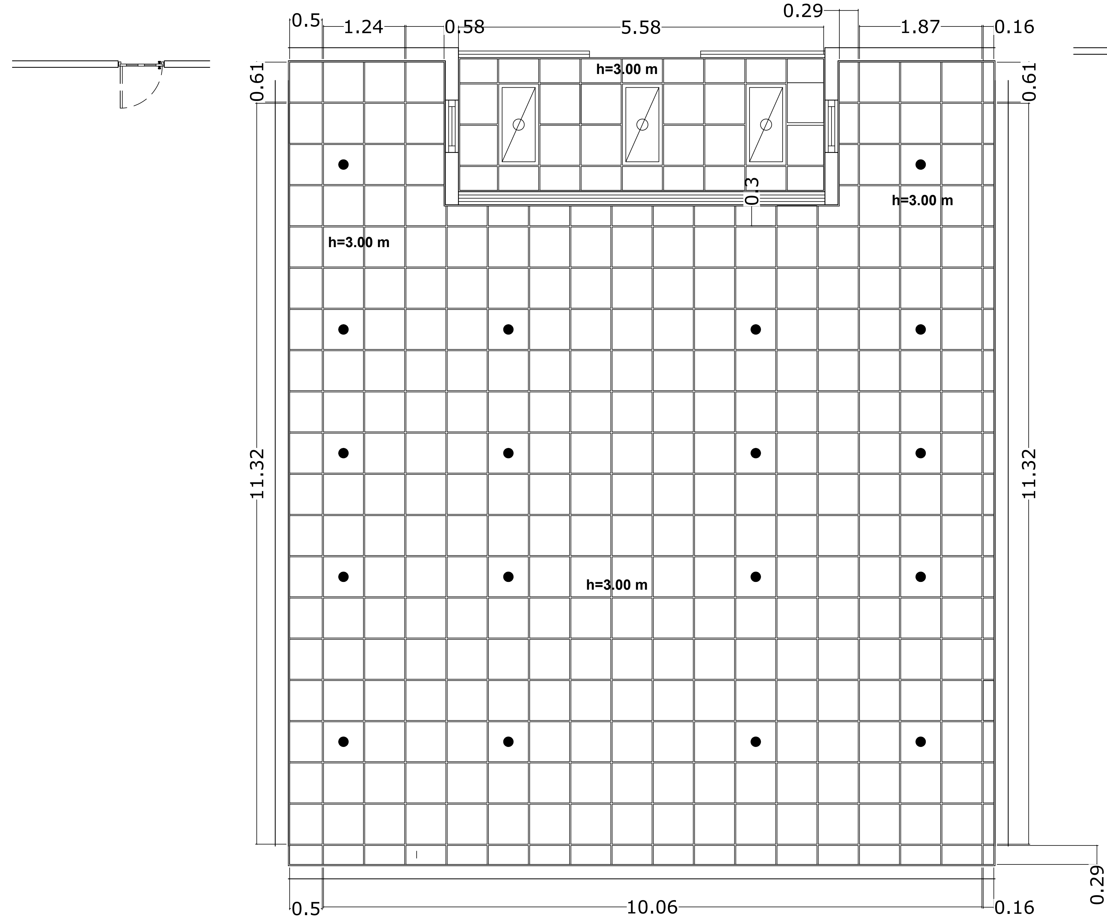
PLANTA PLAFOND PROPUESTA BIBLIOTECA ESCALA: 1:50
