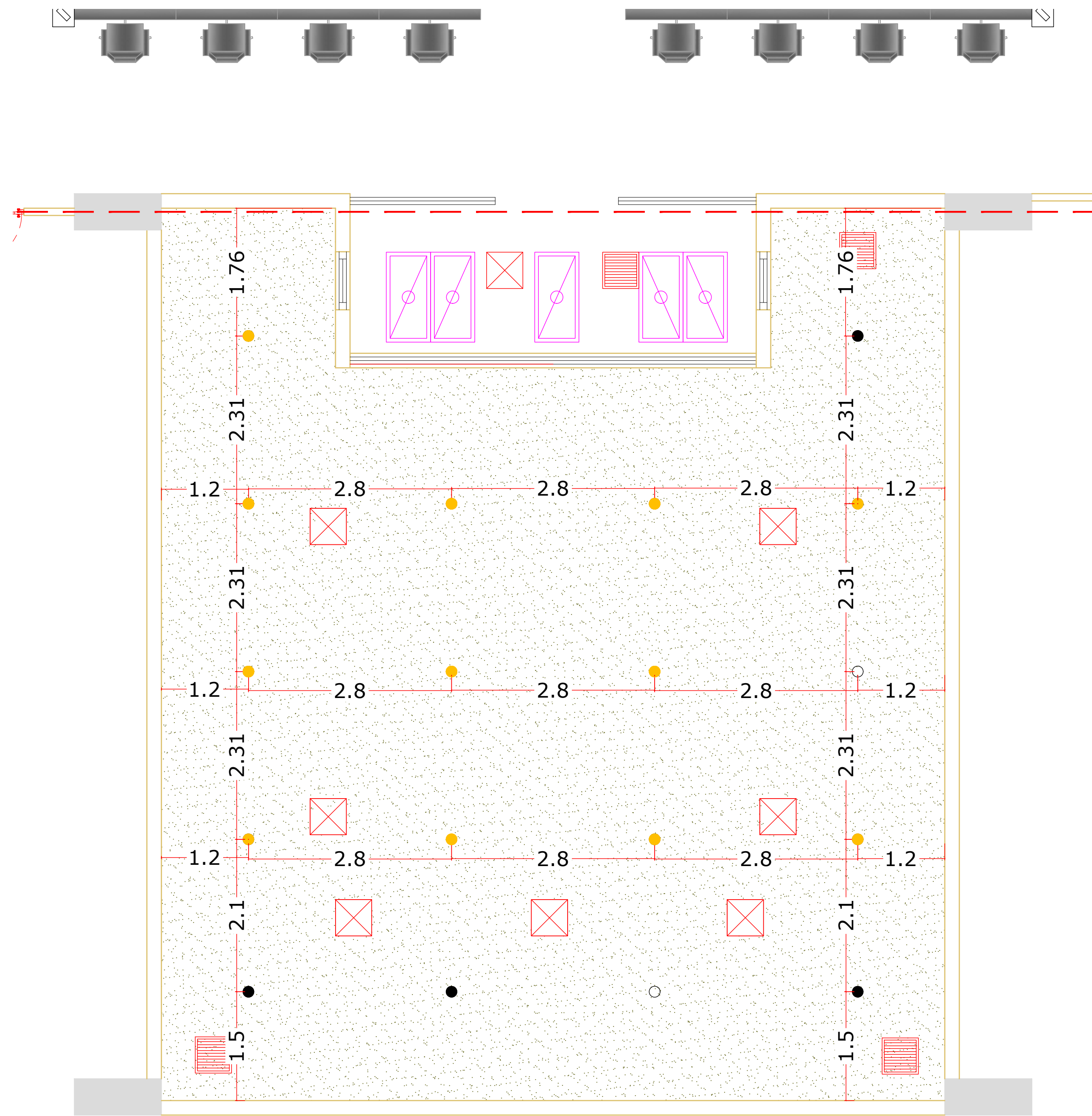
PLANTA DE PLAFONES PROPUESTA BIBLIOTECA NIVEL 3 ESCALA: 1:50
