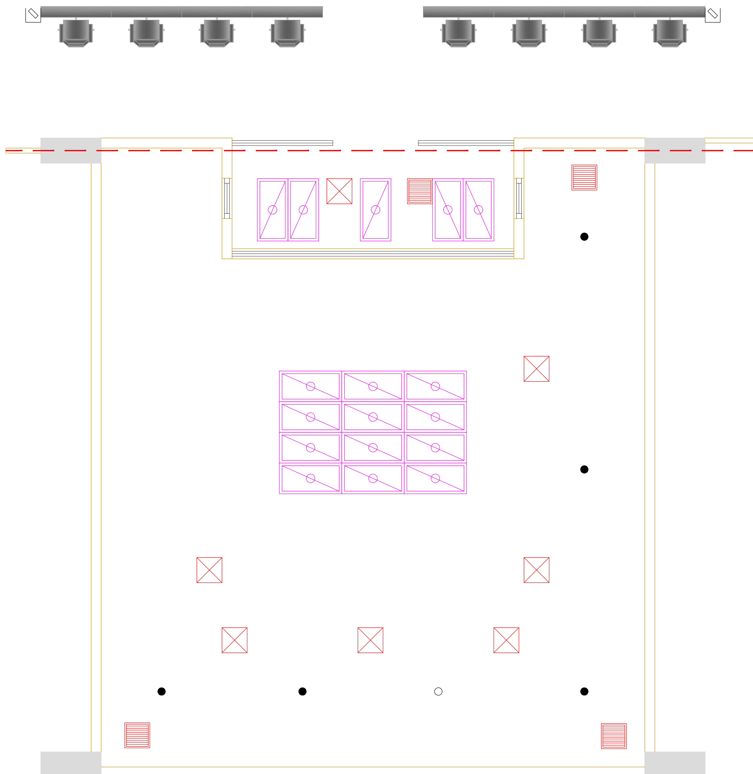
PLANTA DE PLAFONES ACTUAL BIBLIOTECA NIVEL 3 ESCALA: 1:50
