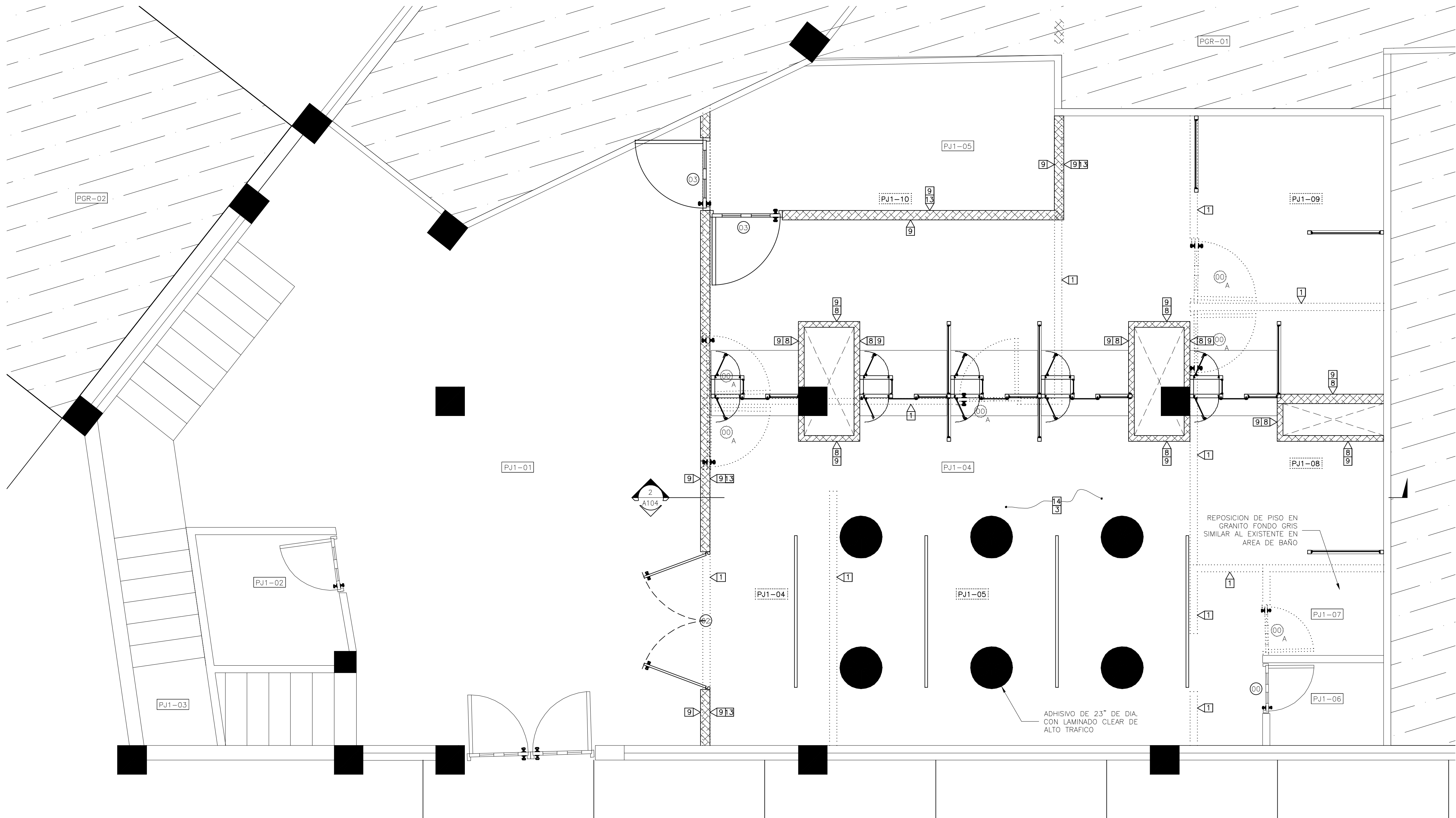
PLANTA DE DEMOLICION Y ADICION SALA DE AUDIENCIA DE ATENCION PERMANENTE ESCALA: 1:33
