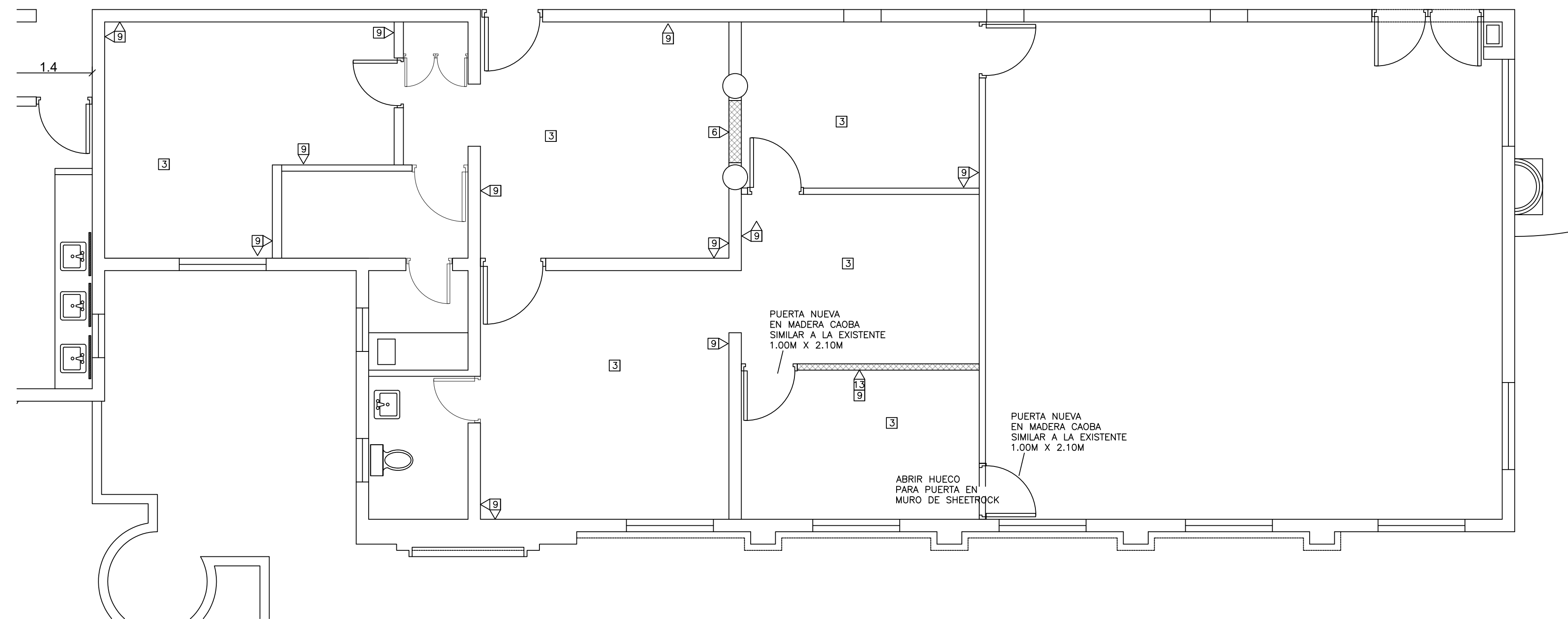
PLANTA DE INTERVENCIONES ESCALA: 1:50
