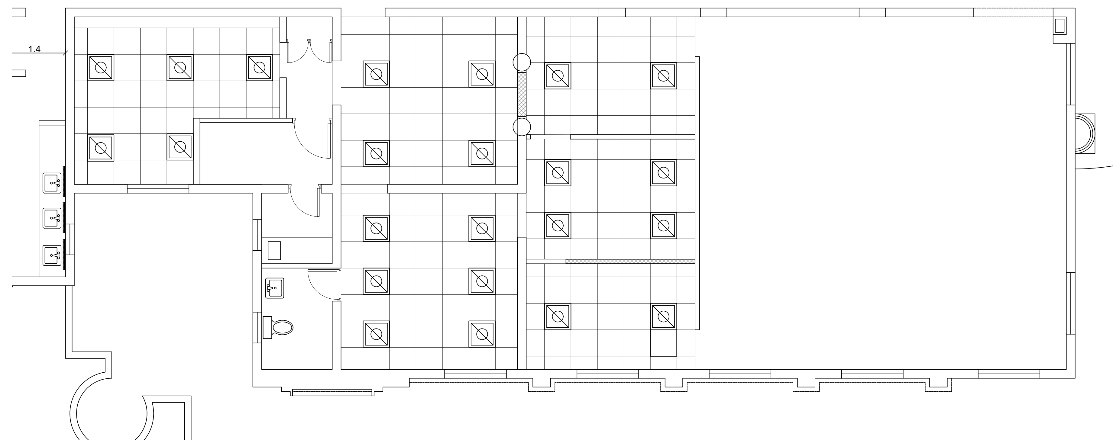
PLANTA DE PLAFONES Y LUMINARIAS ESCALA: 1:50
