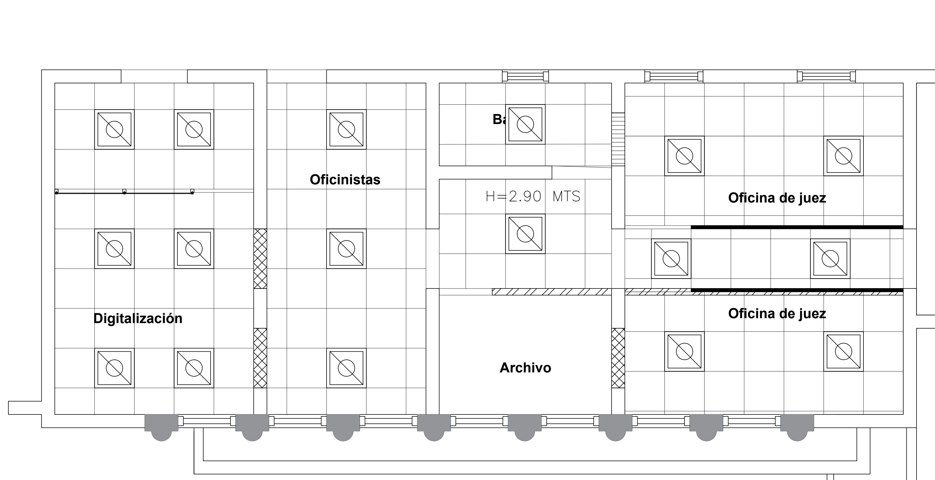
PLANTA DE PLAFONES Y LUMINARIAS
