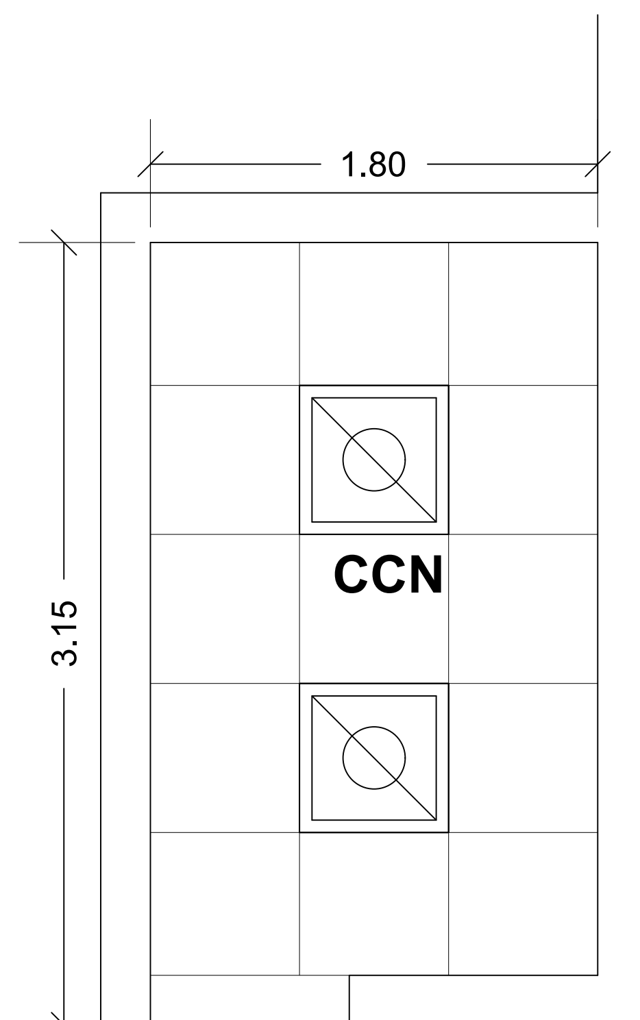
PLANTA DE PLAFONES Y LUMINARIAS CCN
