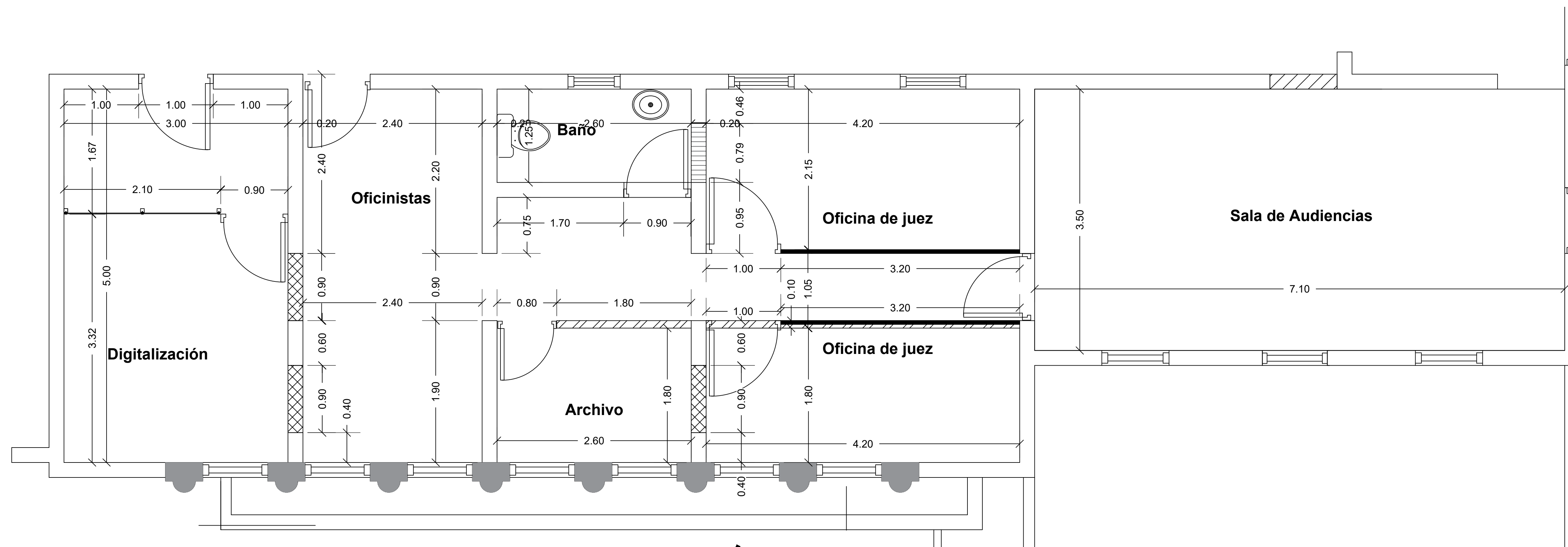
PLANTA ARQUITECTÓNICA DIMENSIONADA
