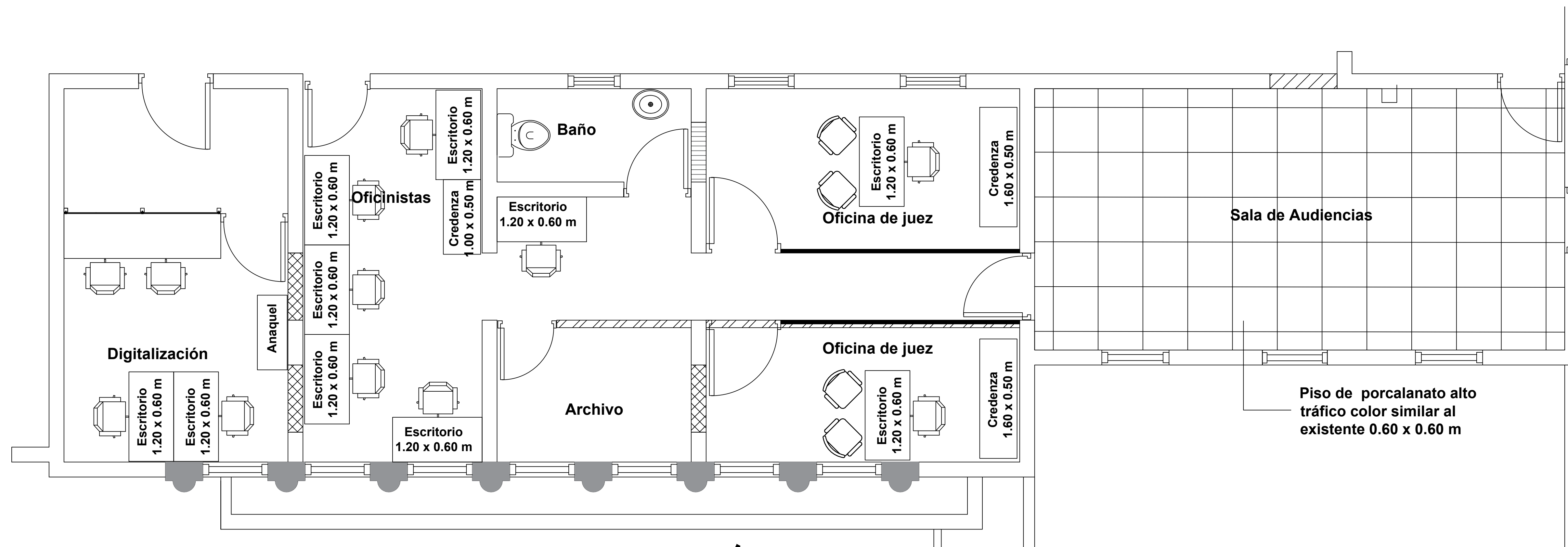
PLANTA ARQUITECTÓNICA PROPUESTA
