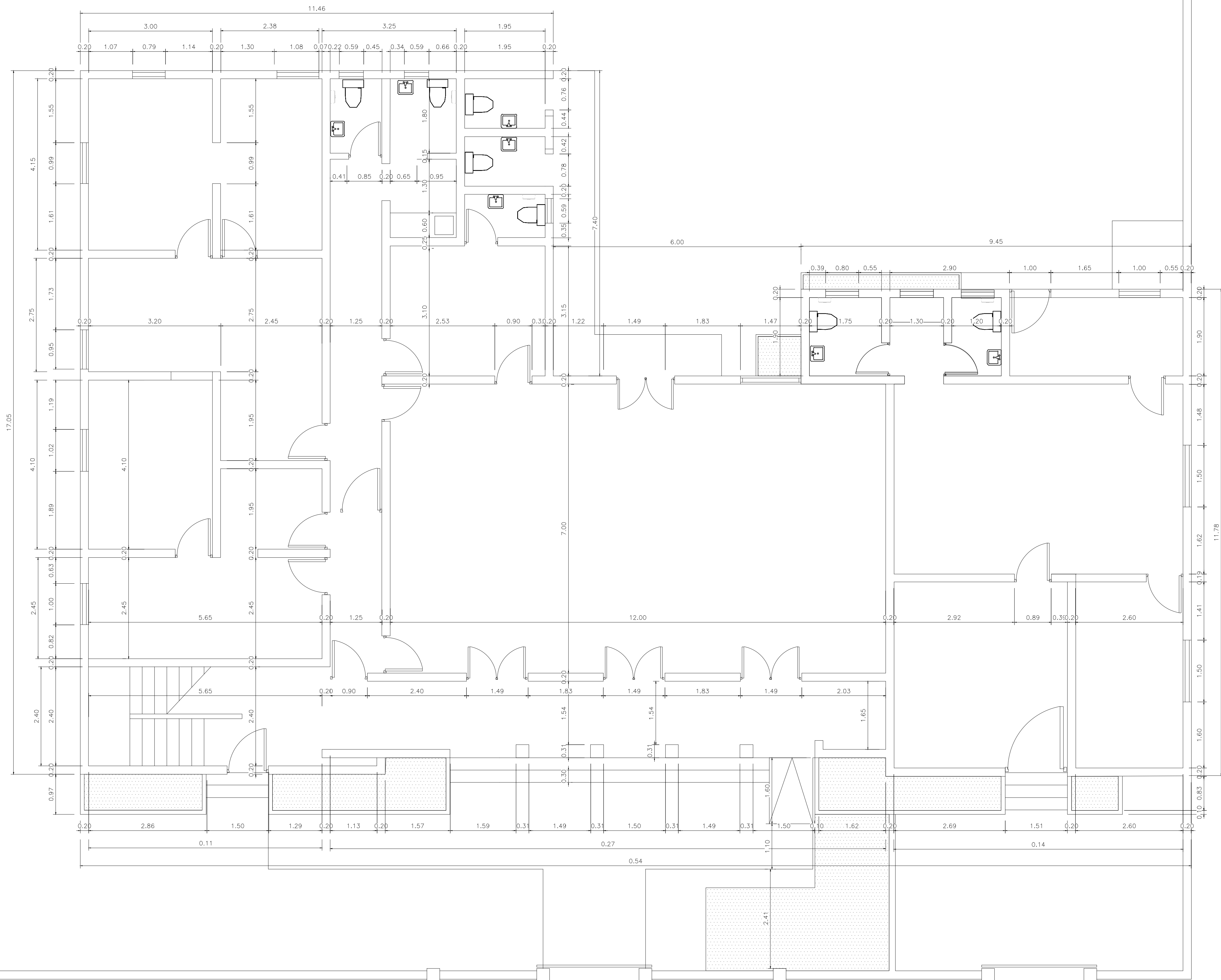
PLANTA DIMENSIONADA EXISTENTE 1ER NIVEL ESCALA: 1:50
