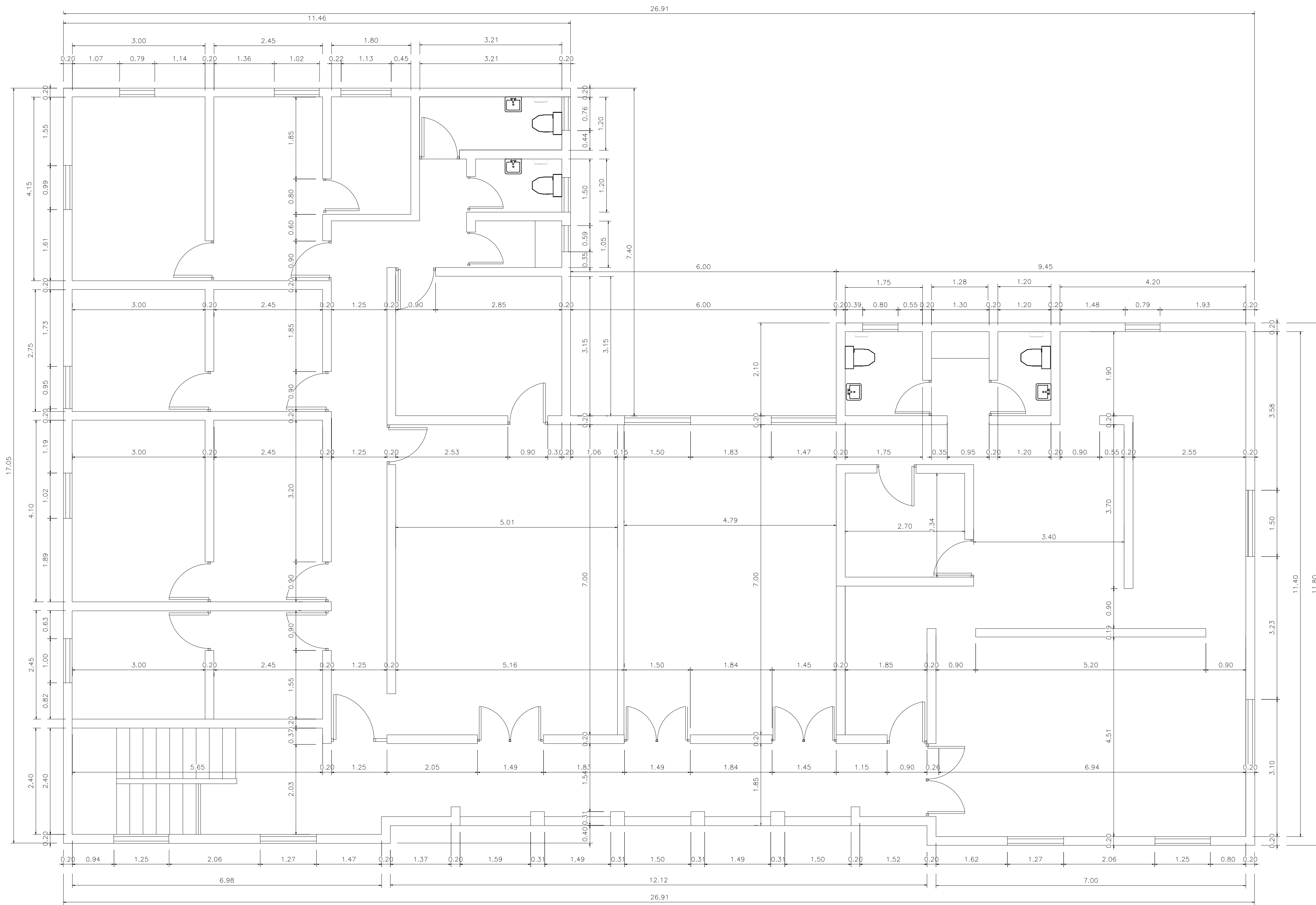
PLANTA DIMENSIONADA EXISTENTE 2DO NIVEL
