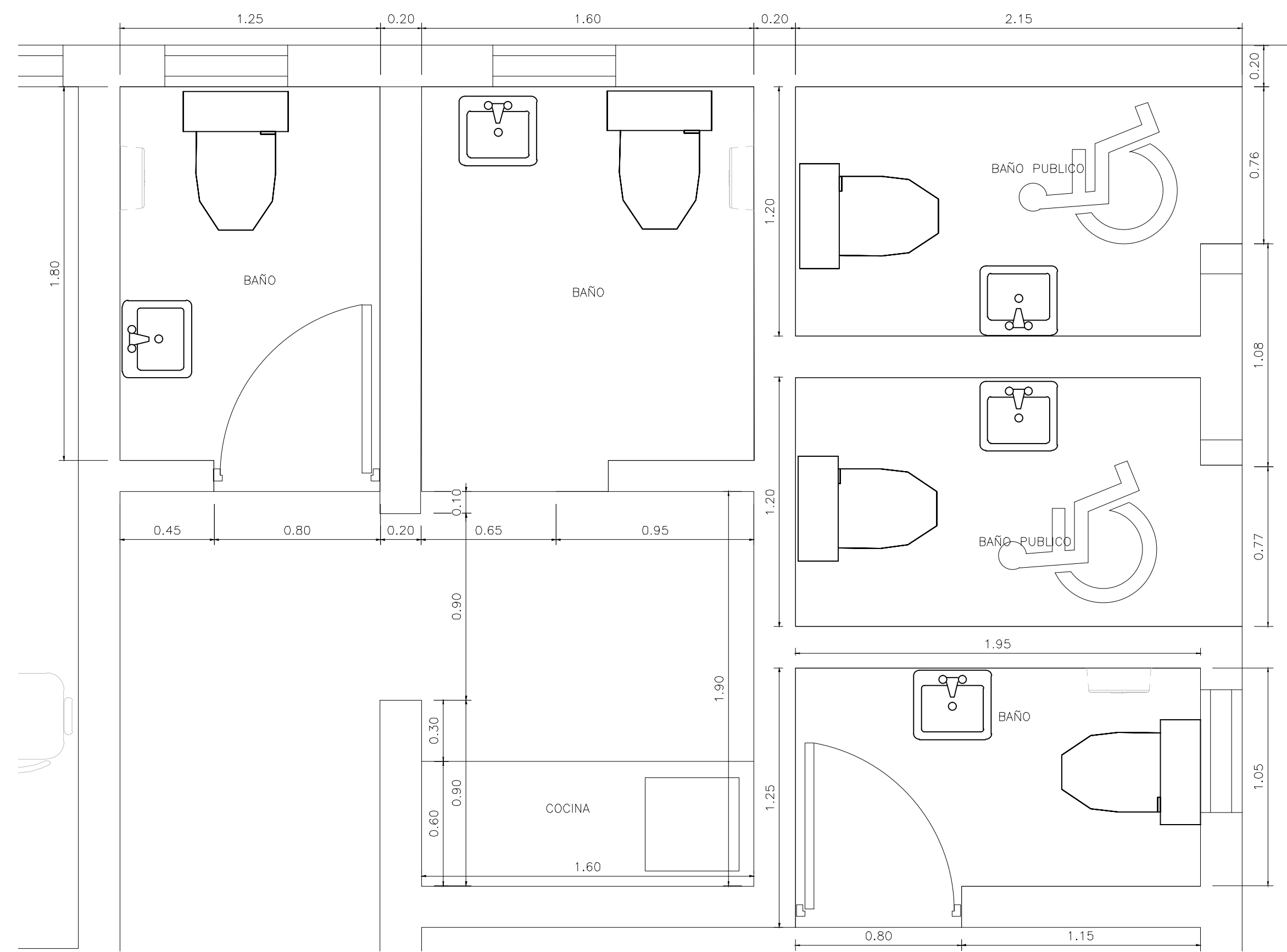
PLANTA EXISTENTE BAÑOS Y COCINAS 1ER NIVEL ESCALA: 1:25
