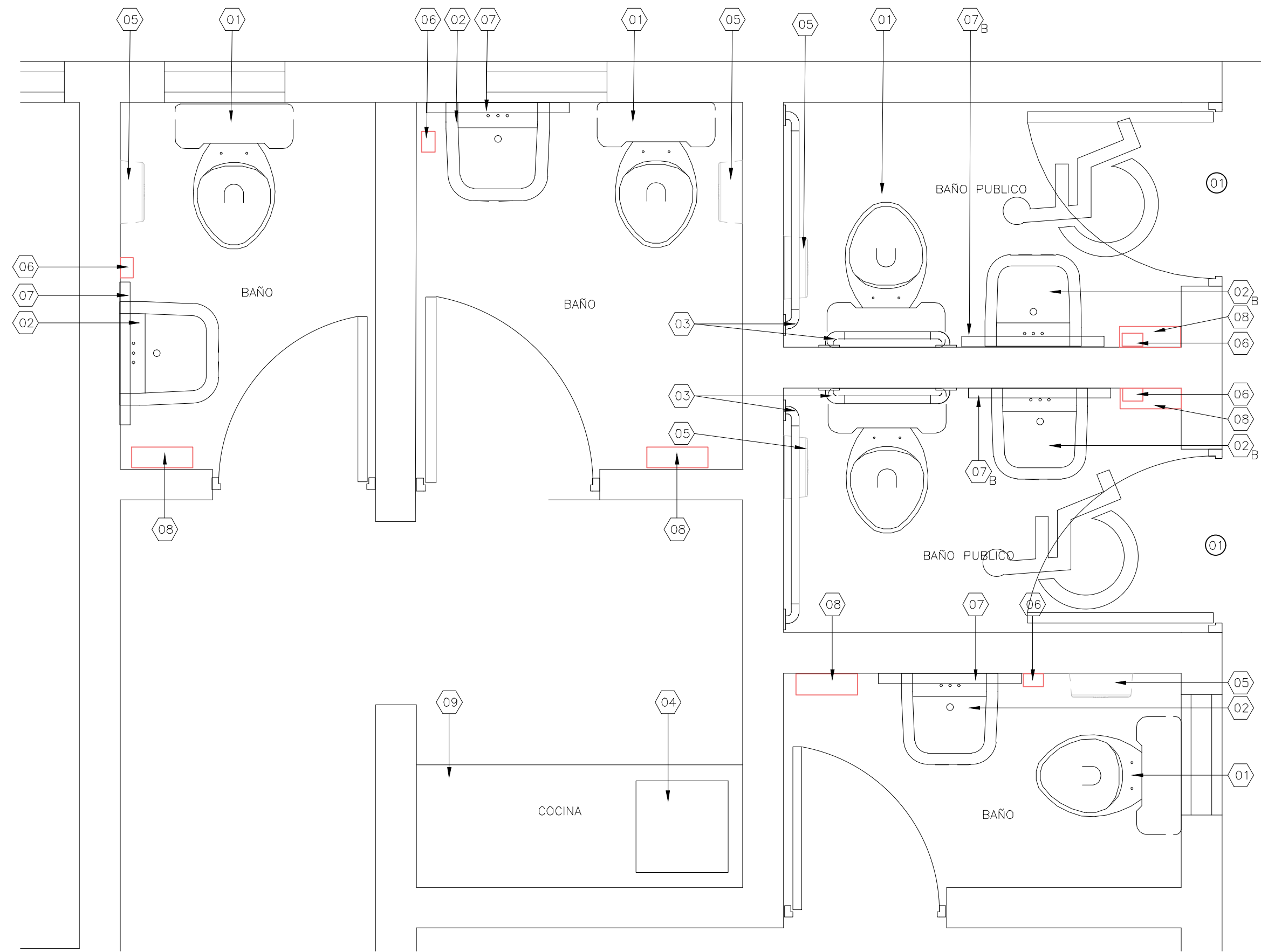
PLANTA PROPUESTA BAÑOS Y COCINAS 1ER NIVEL ESCALA: 1:25
