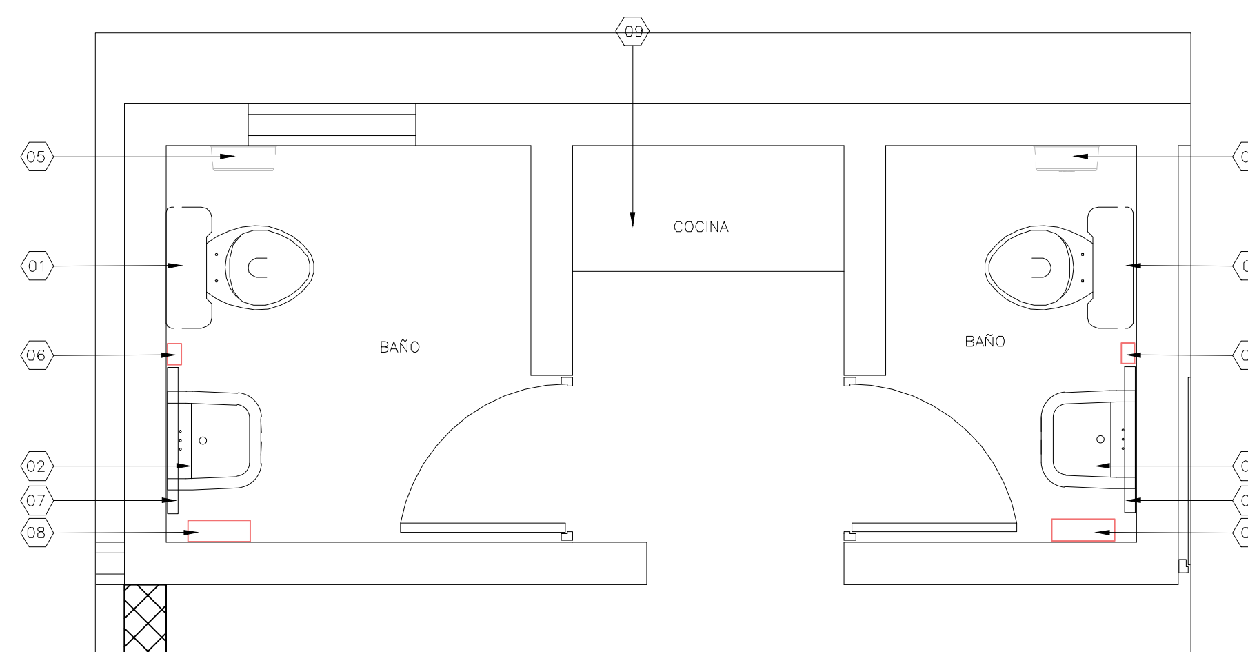
PLANTA EXISTENTE BAÑOS Y COCINAS 2DO NIVEL ESCALA: 1:25
