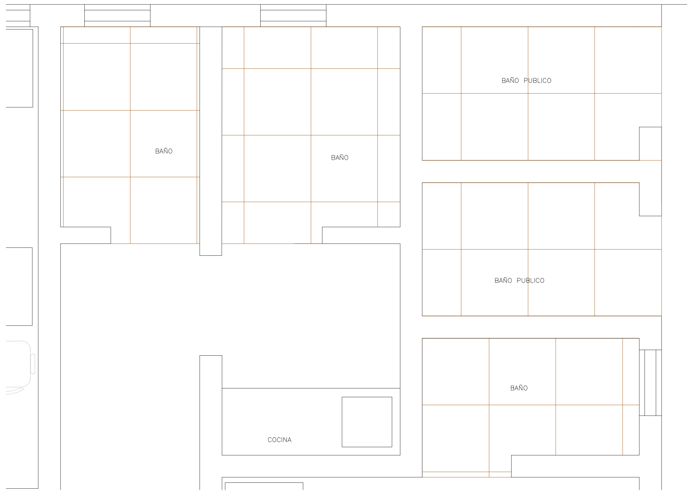
PLANTA DE PISOS ESCALA: 1:25
