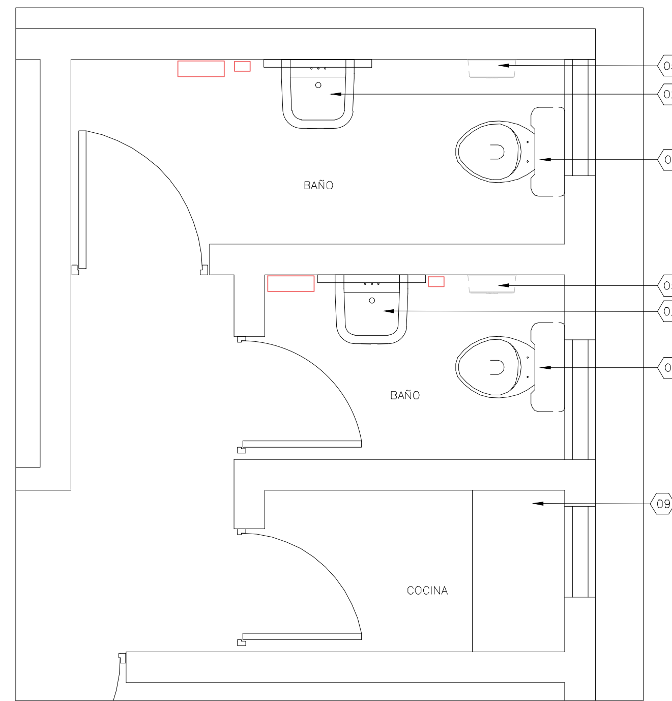
PLANTA PROPUESTA BAÑOS Y COCINAS 2DO NIVEL ESCALA: 1:25
