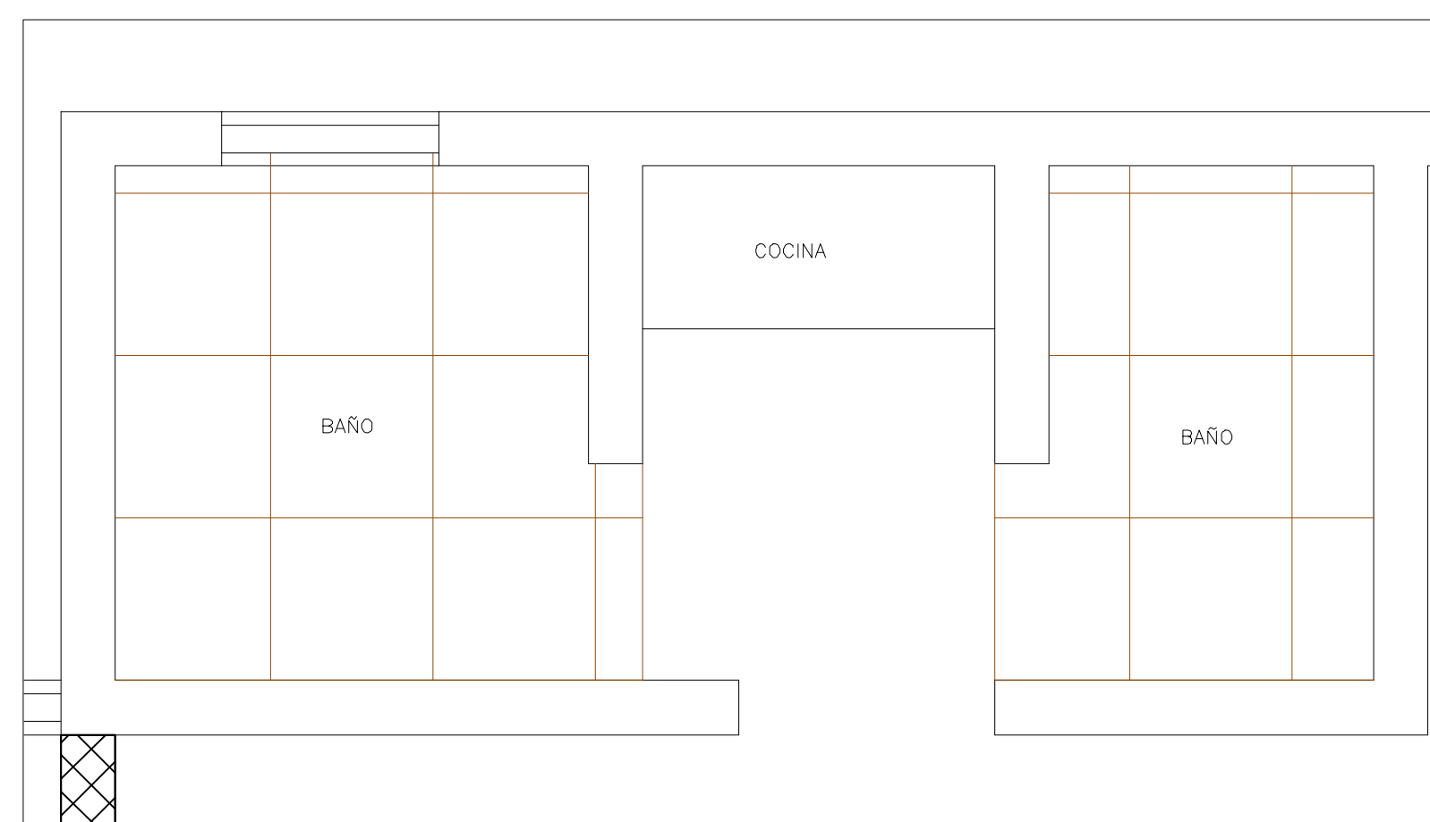
PLANTA EXISTENTE BAÑOS Y COCINAS 2DO NIVEL ESCALA: 1:25
