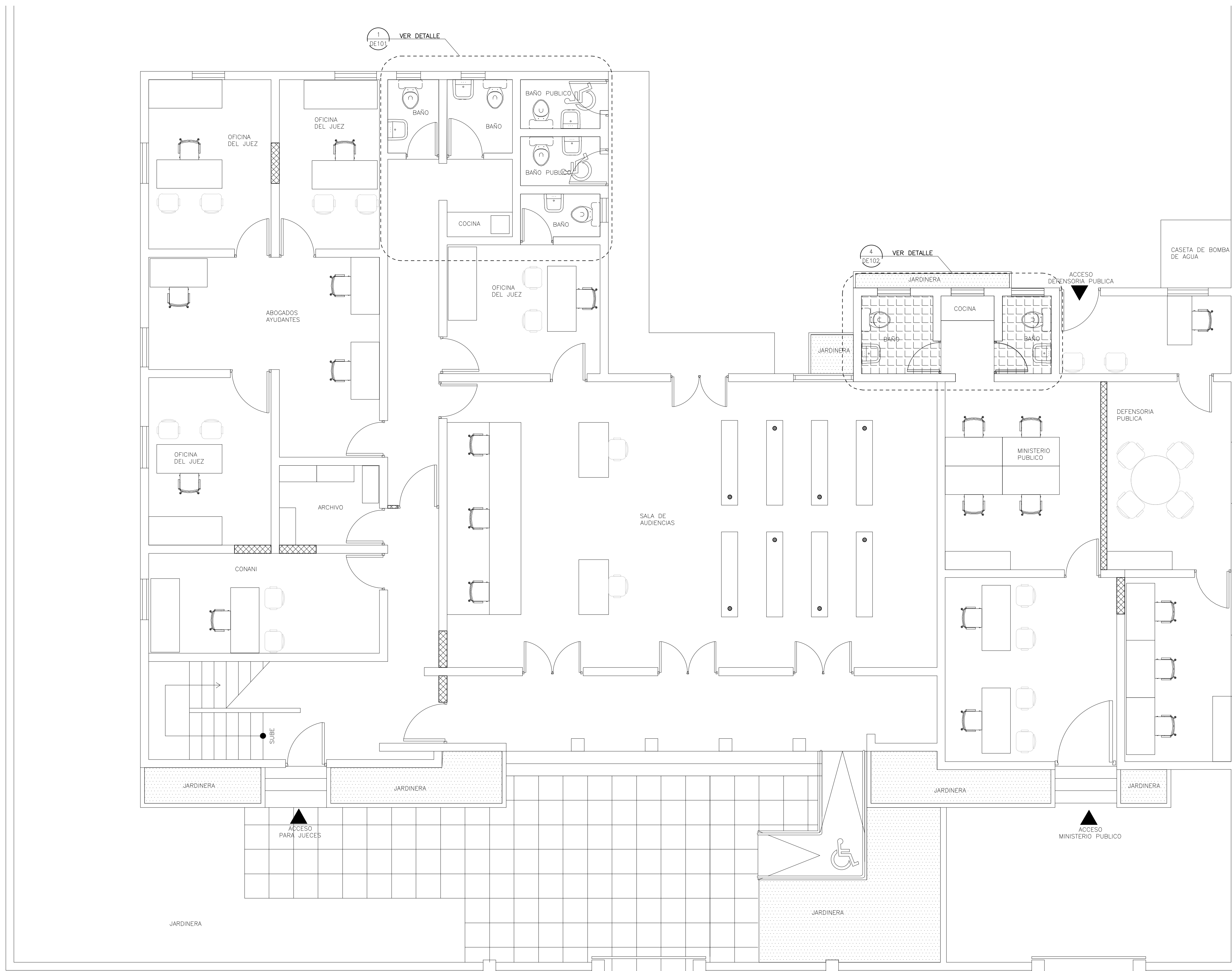
PLANTA ARQUITECTONICA PROPUESTA 1ER NIVEL ESCALA: 1:50
