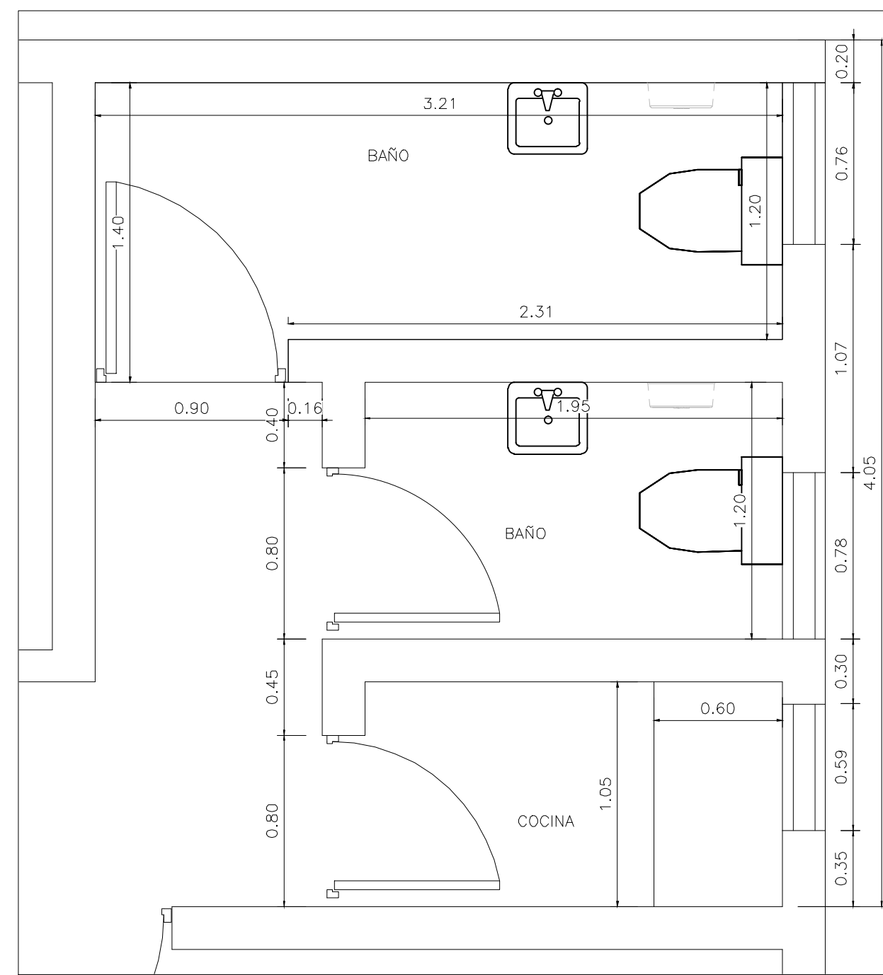
PLANTA EXISTENTE BAÑOS Y COCINAS 2DO NIVEL ESCALA: 1:25
