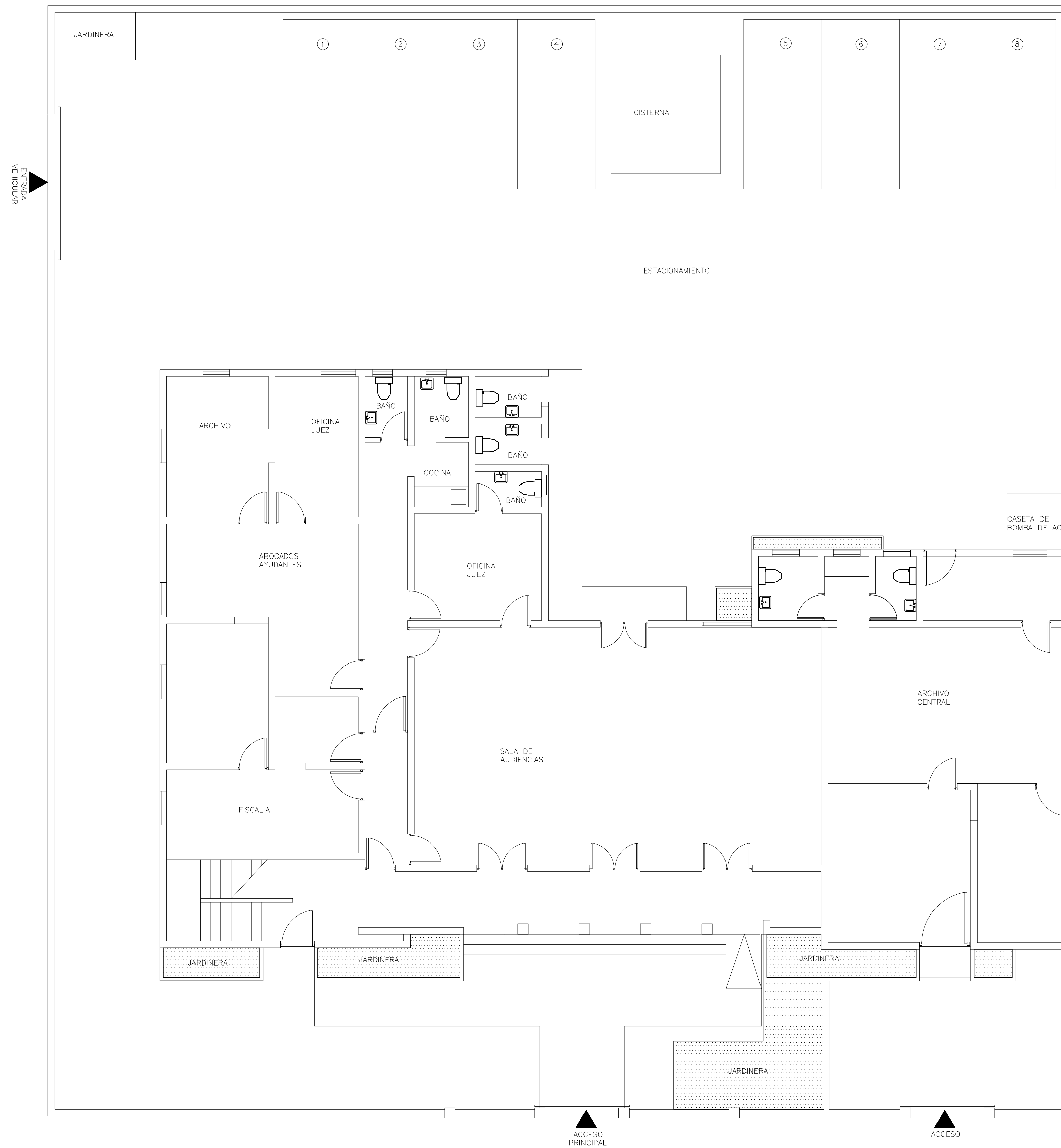
PLANTA ARQUITECTONICA DE CONJUNTO EXISTENTE 1ER NIVEL ESCALA: 1:75
