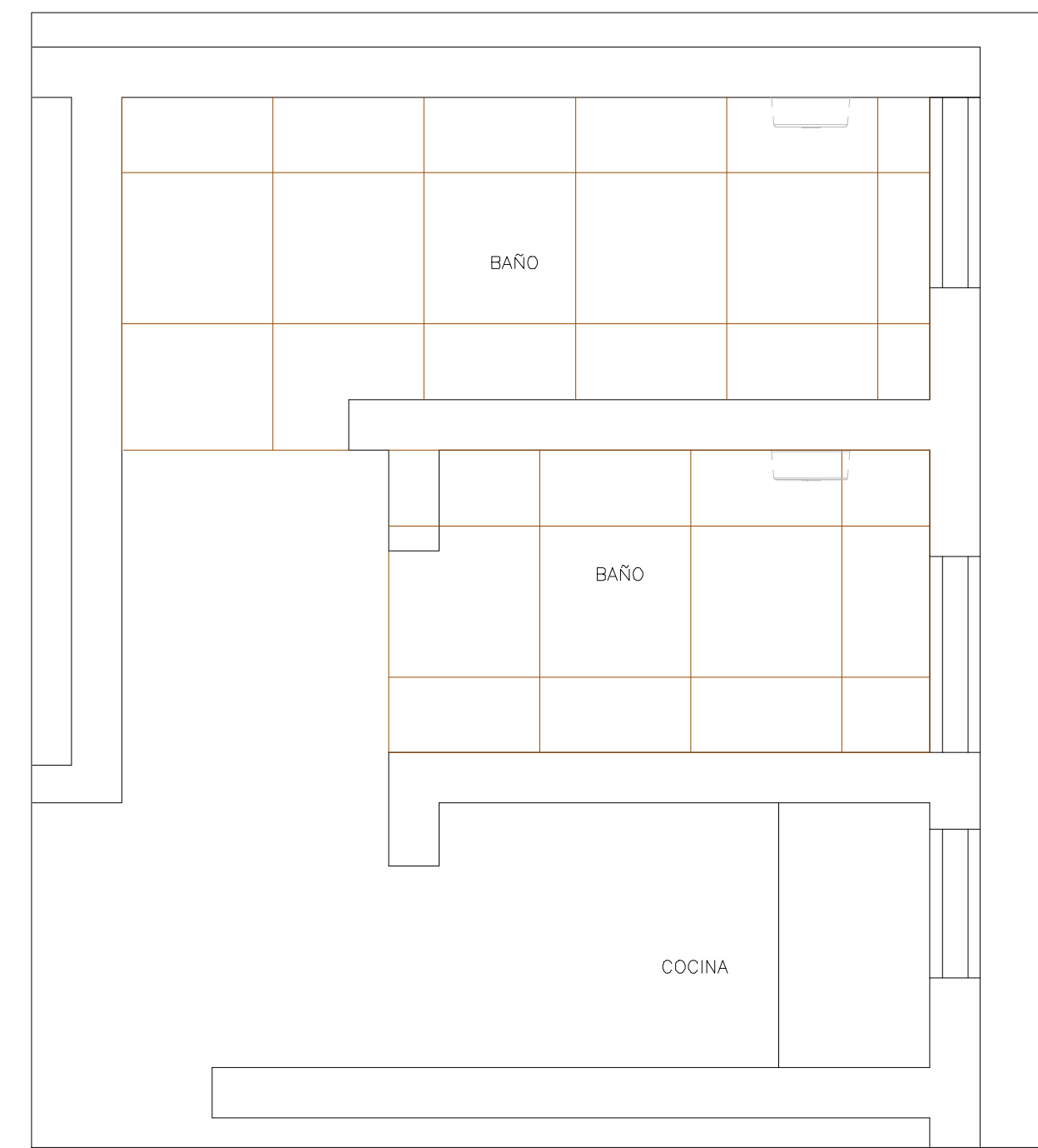
PLANTA DE PISOS DE BAÑOS 2DO NIVEL ESCALA: 1:25
