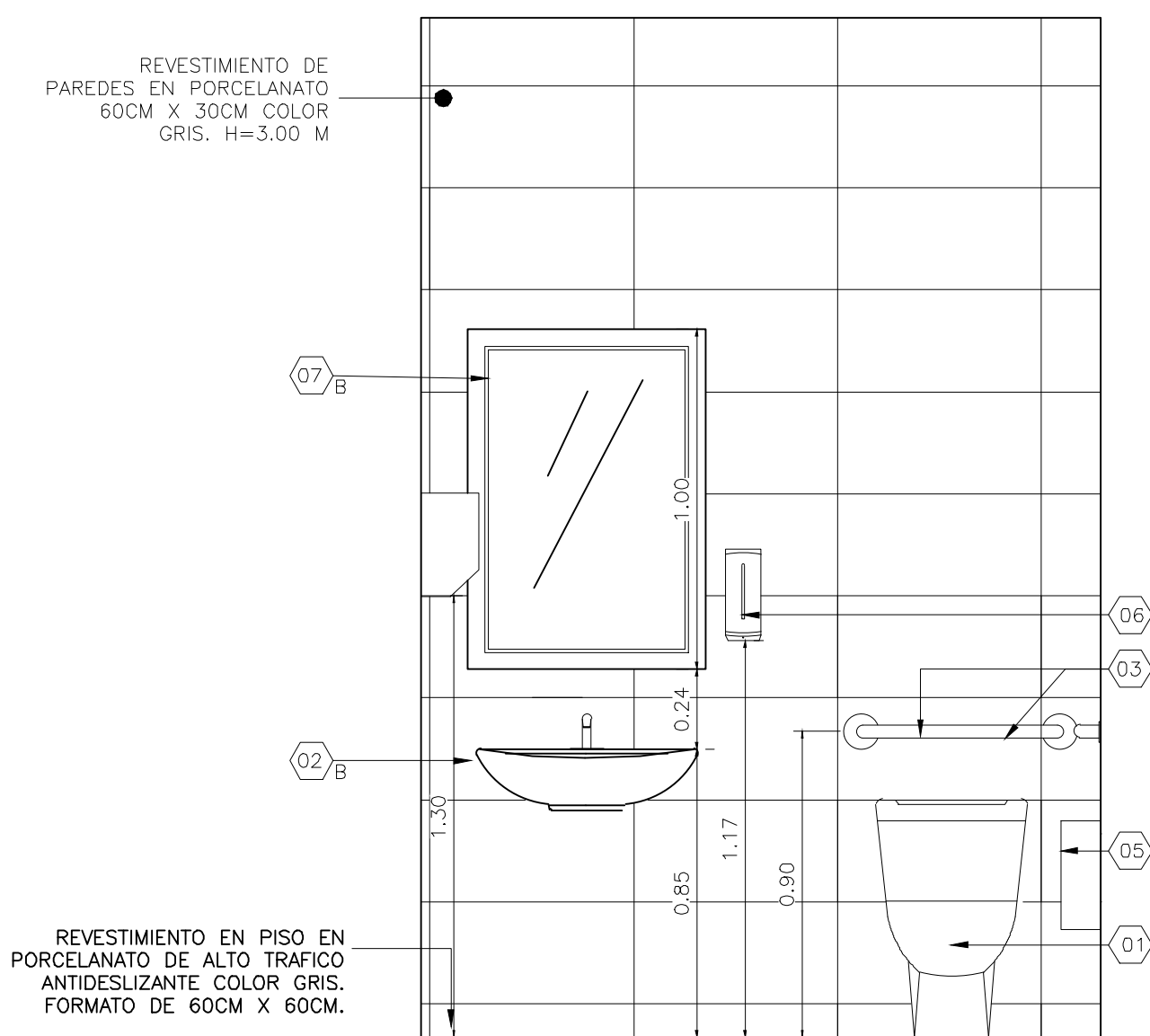
ELEVACION TIPICA PARA BAÑOS ACCESIBLES ESCALA: 1:20
